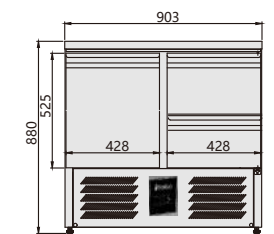
GTS-S901 S/S Top 2×GN1/2
