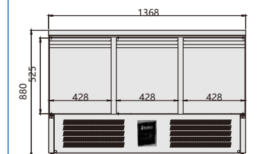
GTS-S903 S/S Top
