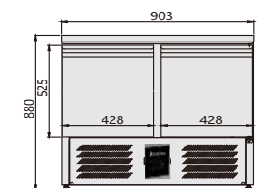
GTS-S901 S/S Top 2×GN1/2
